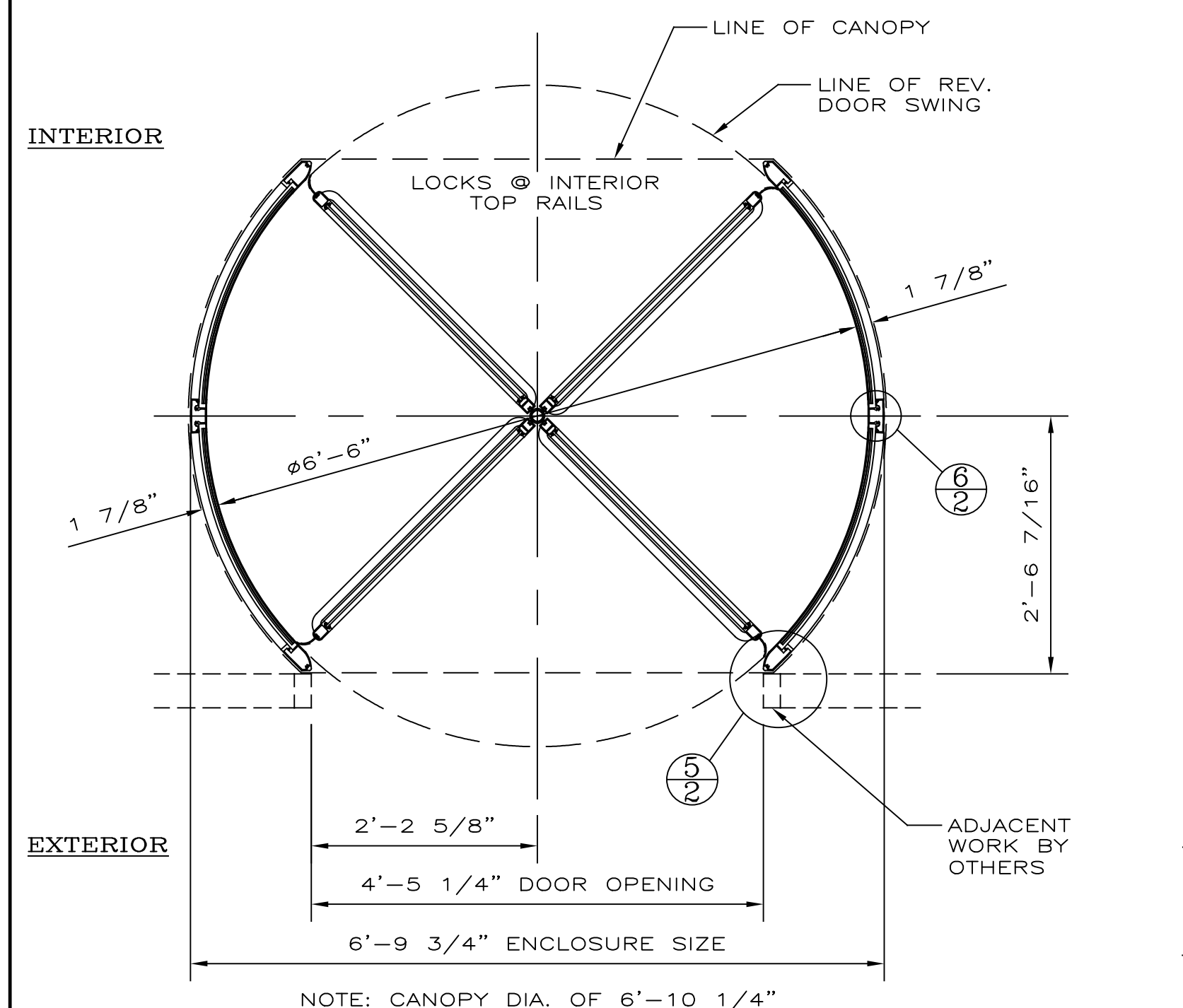
PLAN SCALE: 3/4" = 1'-0"
